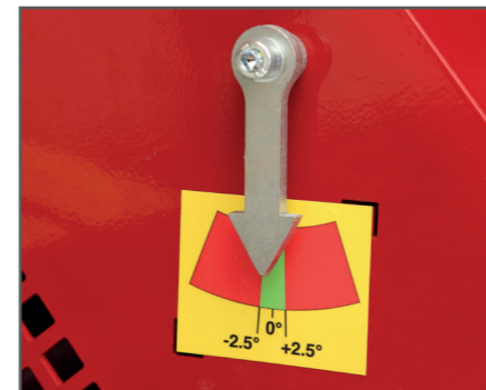
Anzeige Maschinenneigung
