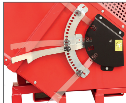
Die Schnittlängeneinstellung von 250 - 520 mm ist einfach ohne Werkzeug möglich. Es ist kein Trommelwechsel notwendig.
